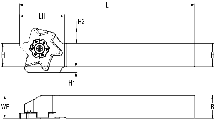
本图为右手刀杆 (R)
