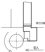
· Y-SVJC型 (外径加工)
