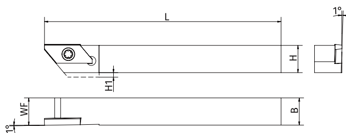
●本图为右手刀杆(R)
