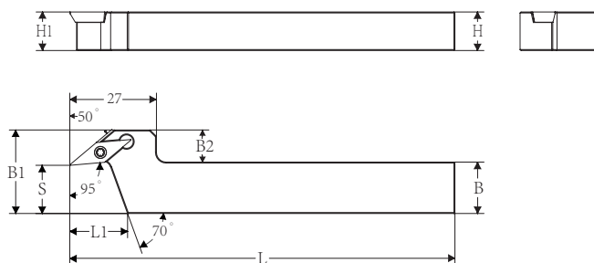
· 本图为右手刀杆
