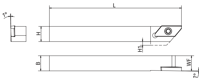
●本图为左手刀杆(L)
