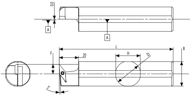
本图为左手刀杆 (L)
