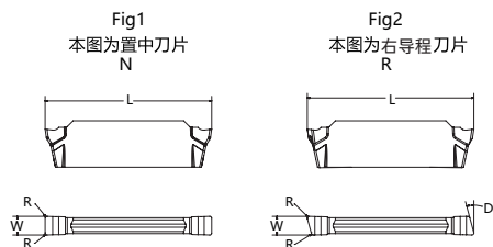
刀片示意图
