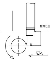
· Y-SDNCN型 (外径加工)
