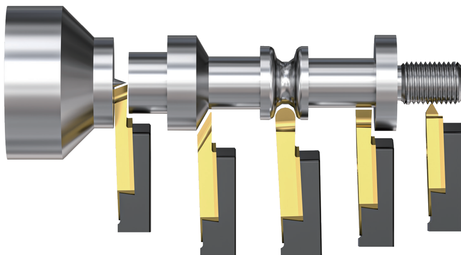
切断 后扫 仿型 切槽 螺纹 最大切断直径 \Phi 12\text{mm}
