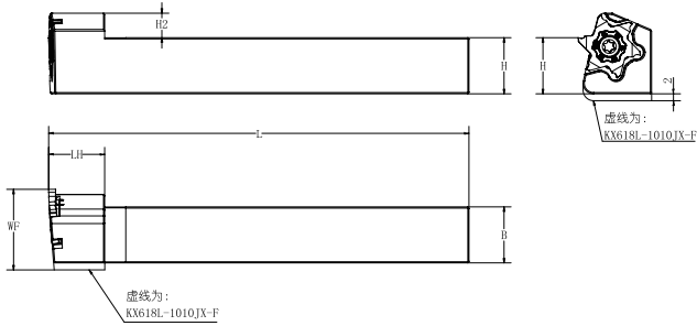
本图为左手刀杆 (L) 左手 (L) 刀杆适用右手 (R) 刀片
