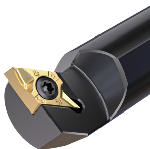
·KDC-SDUX型 (副主轴外径/端面加工)
