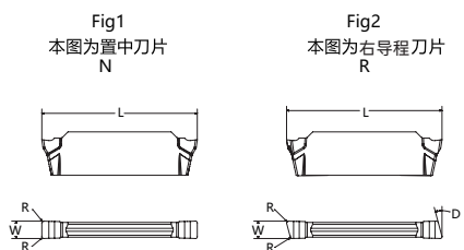
刀片示意图
