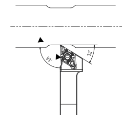
· 加工示意图
