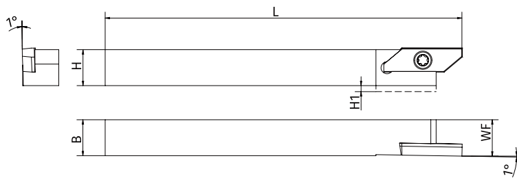
●本图为左手刀杆(L)
