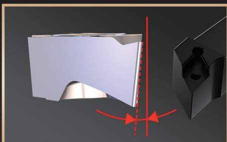
② 刀片自带后角
