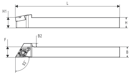
· 本图为右手刀杆
