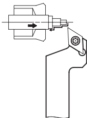
· 加工示意图
