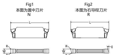
刀片示意图
